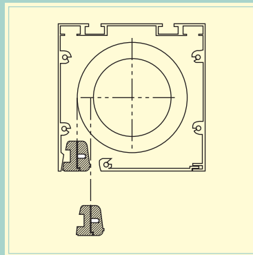
Screen Case-Profil
